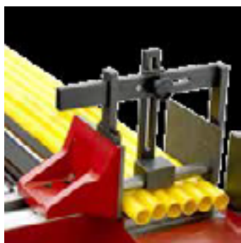
Mechanische bundelklemming
