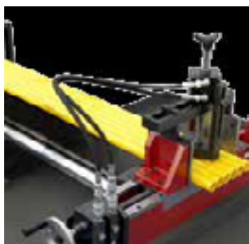
Hydraulische bundelklemming
